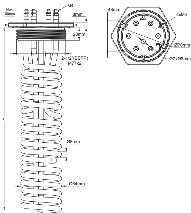
带2½" BSPP 和M77×2接头
